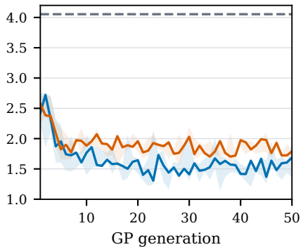
MMAS
